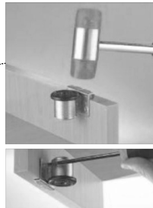
Montaż regulatora poziomu
